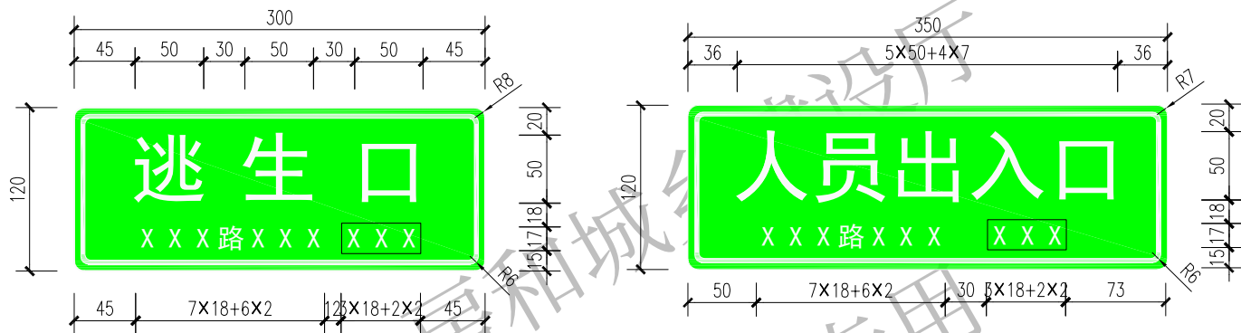
逃生口、人员出入口标识 1:5
