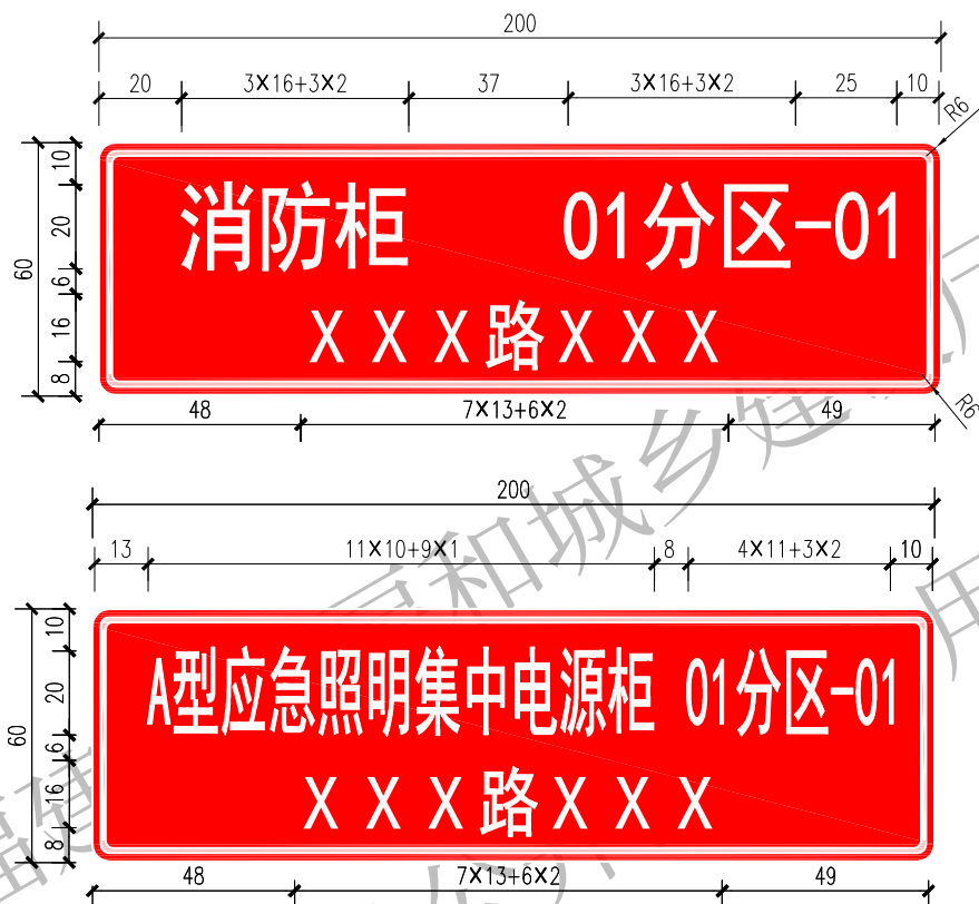
机柜标识 1:4
