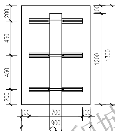
立面图 1:30
