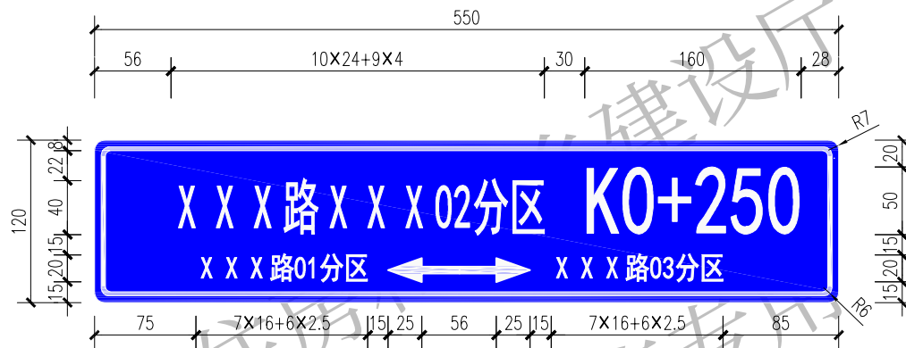
综合管廊里程标识 1:5
