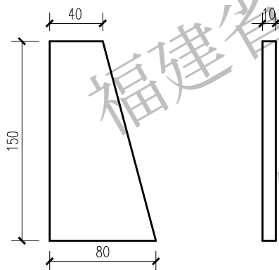
底座加劲筋 1:4
