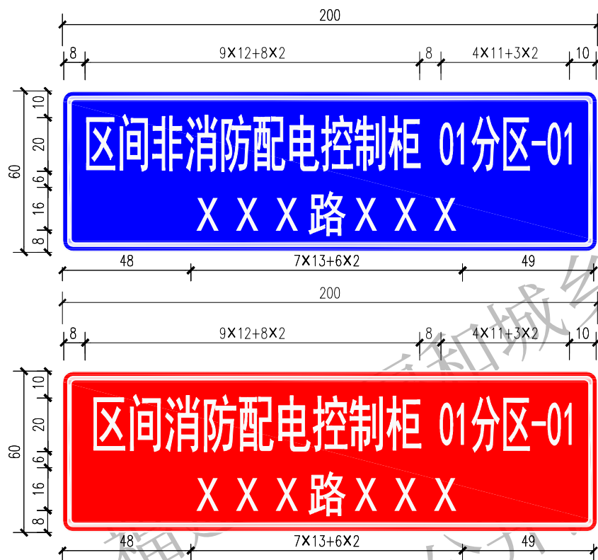
机柜标识 1:4
