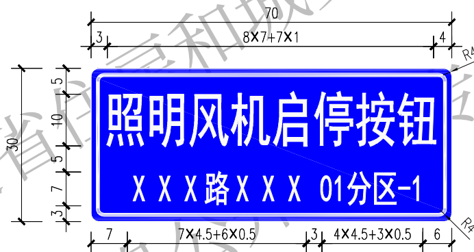
启停按钮标识 1:4
