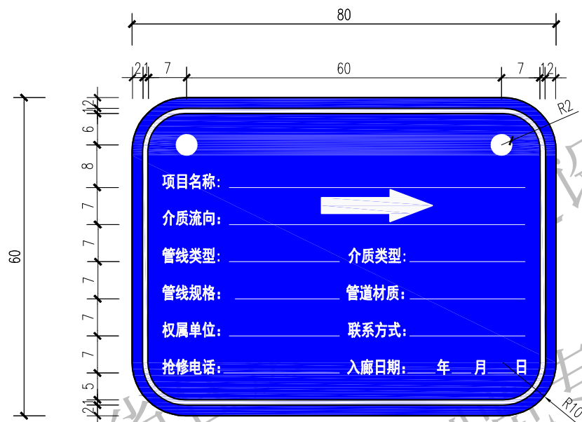
管道铭牌标识 1:1
