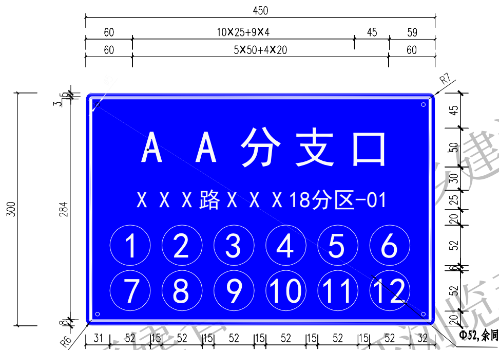
管线分支口标识 1:5
