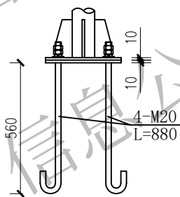
底座连接大样 1:20
