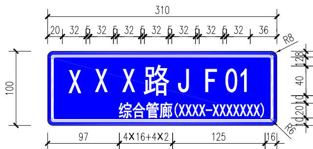
外部进风口标志 1:5
