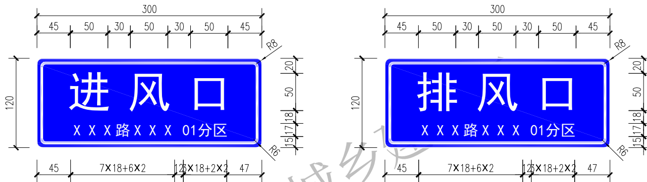
进风口位置标识 1:5
