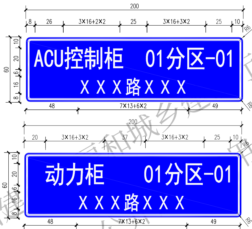
机柜标识 1:4
