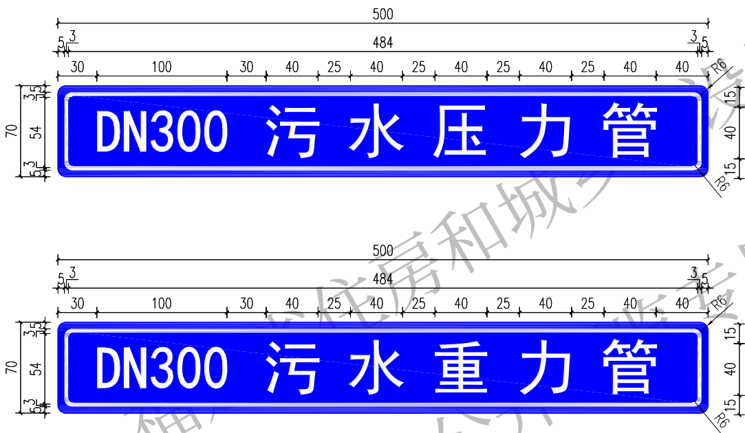
管道标识 1:4
