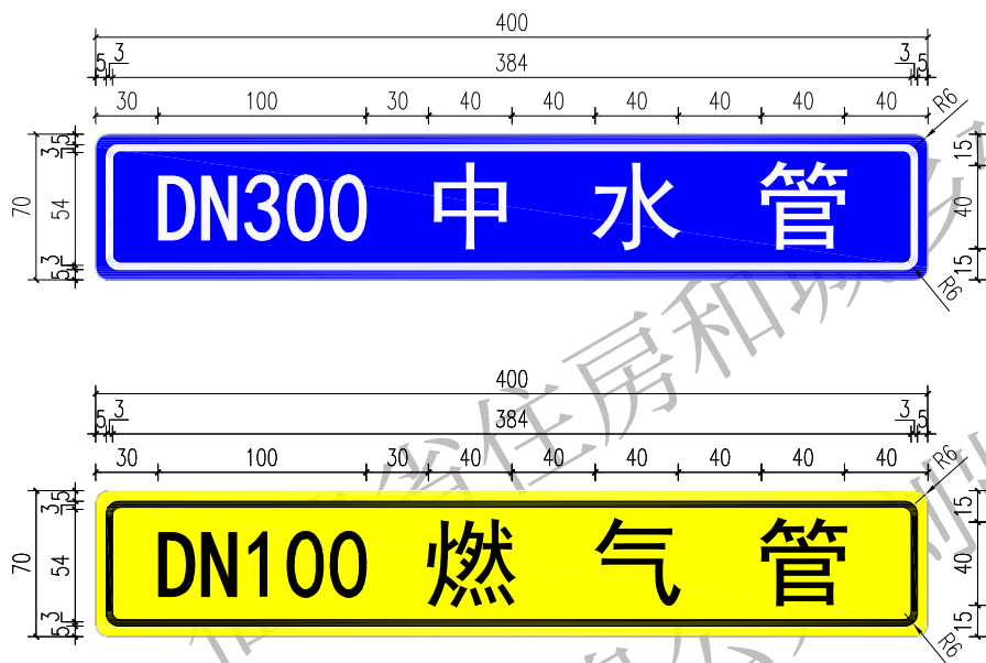
管道标识 1:4
