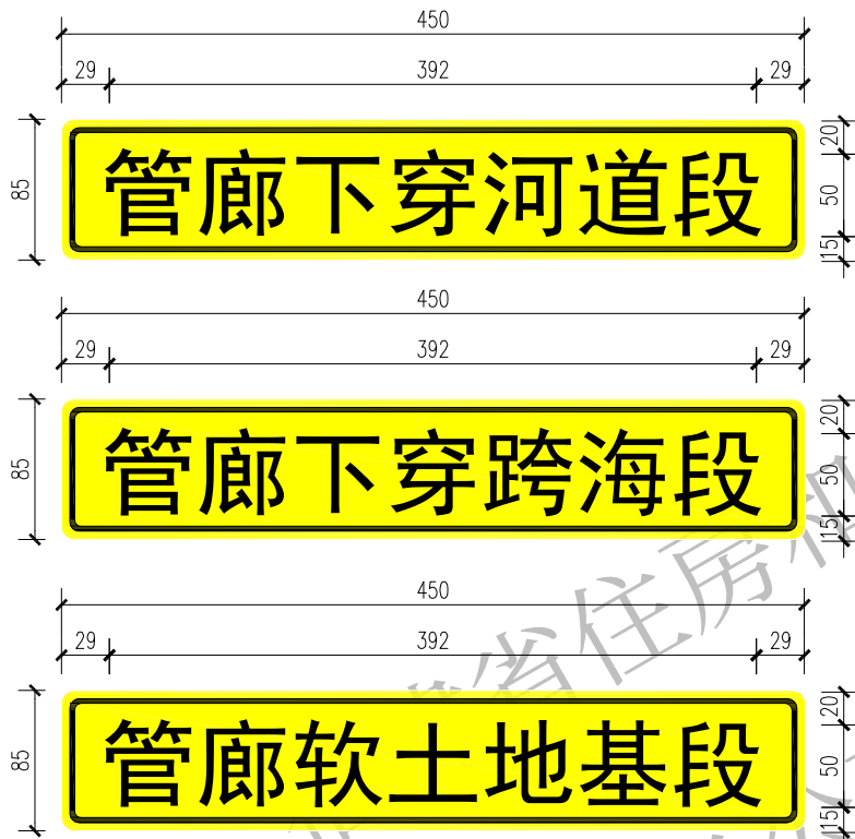
管廊下穿标识 1:5
