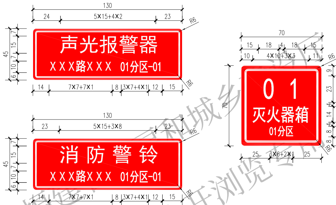
消防报警标识 1:4
