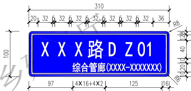
外部吊装口标志 1:5
