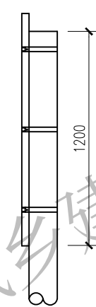
侧面图 1:30
