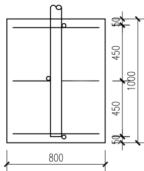
基础纵剖面 1:30
