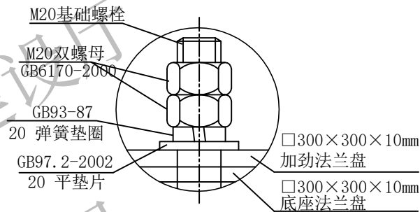
A局部放大 1:2
