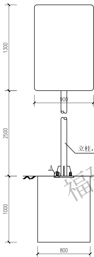
标志立面图 1:30
