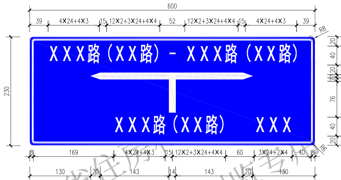
管廊交叉口预告标识 1:5
