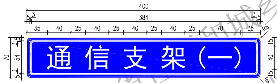
支架标识 1:4
