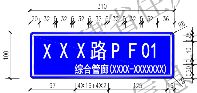
外部排风口标志 1:5
