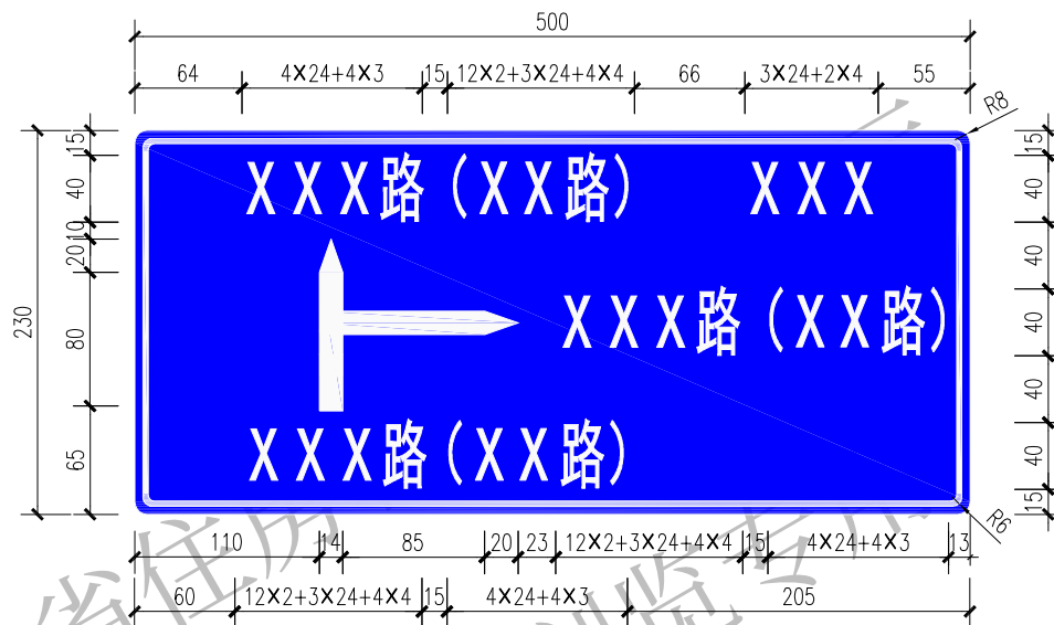
管廊交叉口预告标识 1:5
