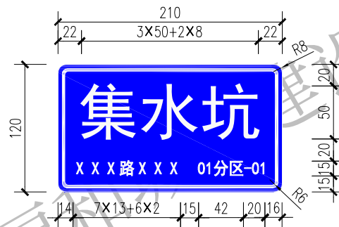
集水坑位置标识 1:5
